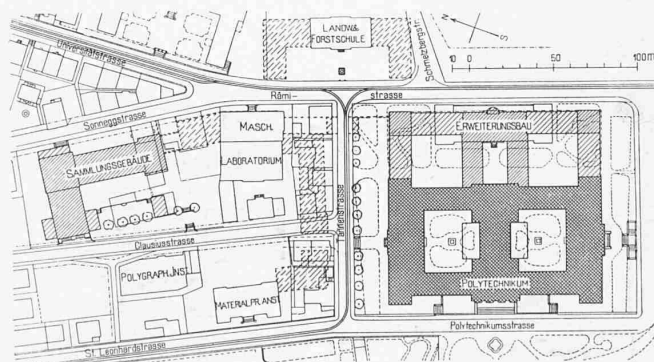
Lageplan 1:4000
