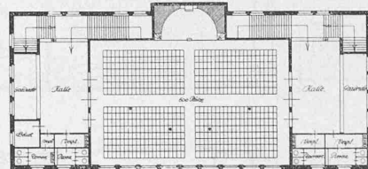
Grundrisse vom Obergeschoss und Dachgeschoss. — 1:800.
