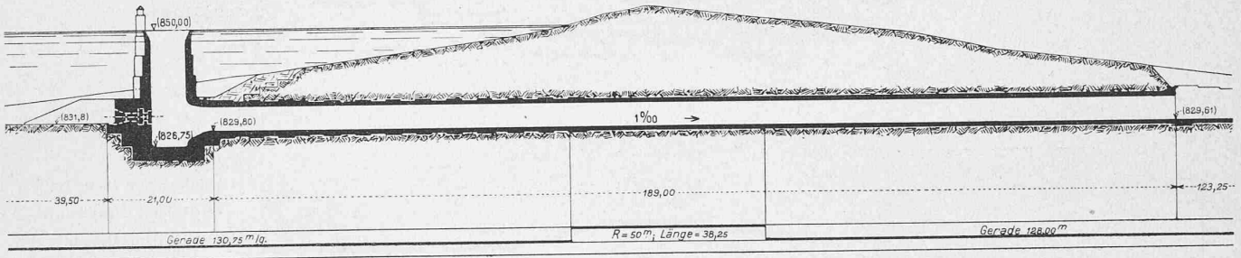
Abb. 17. Längsschnitt durch Grundablass und Ueberlauf-turm und den Ablauf-tunnel nach dem Löntsch. — Masstab 1 : 1200.
