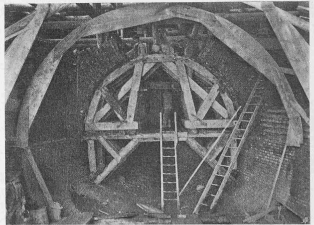
Abb. 31. Zimmerung und Mauerung des Ablaufsturms (10. April 1908).
