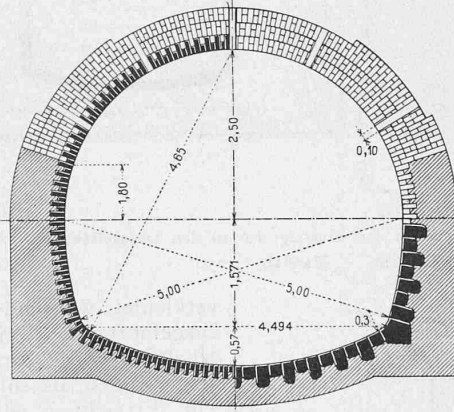
Abb. 29. Profil des Ablaufsturms. — 1 : 100. Links: oberer Teil; rechts: unterer Teil.
