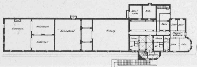
Grundrisse vom Erdgeschoss (Seite 224) und vom Kellergeschoss und Obergeschoss (Seite 225). — Masstab 1: 800.
