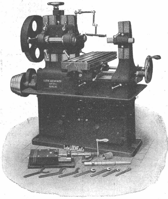
Selbsttätige Fräsmaschine mit vertikaler Spindelbewegung Nr. 13 I.
