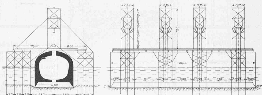
Abb. 5. Gerüst-Schema für die Versenkung der Seine-Caissons. — Masstab 1:500.
