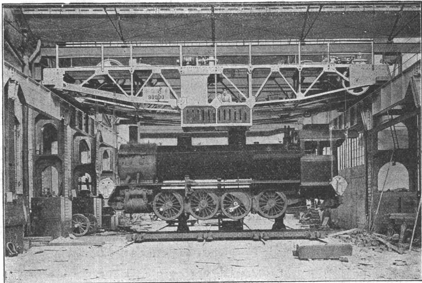
Elektrisch betriebener Lokomotivhebekran, 90 000 kg Tragfähigkeit, 12,6 m Spannweite. Stettiner Maschinenbau-A.-G. „Vulkan“, Stettin.
