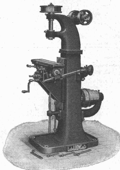
Vertikale Fräsmaschine Nr. 16 Mod. O.
