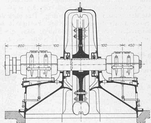
Abb. 22. Grundriss und Schnitte der 5500 PS-Pelton-turbine (mit Handregulierung der Nadel) der Zentrale Ackersand. Gebaut von Piccard, Pictet &amp; Cie. in Genf. — 1 : 50.
