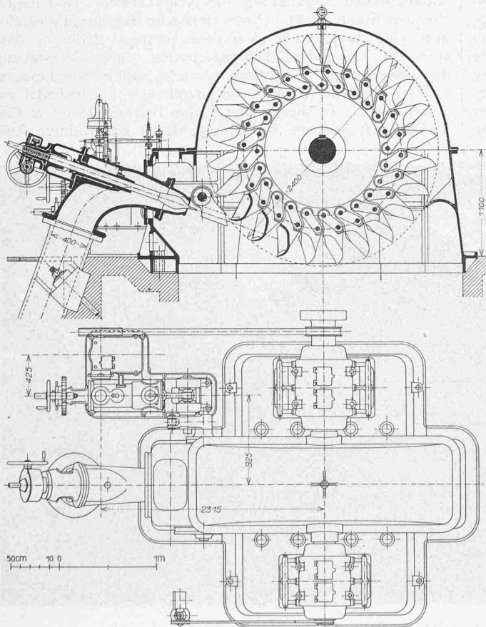
Abb. 25 und 26. Schnitt und Ansicht der automatischen Nadel-Regulierung. — 1 : 50.
