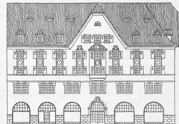
Fassade des Gebäudelflügels an der Poststrasse. — 1:400.
