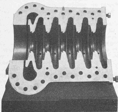
Abb. 6. Gegossene Gehäusenhälfte der Pumpe in Abb. 4.
