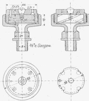
Abb. 9. Sulzersche Streudüse. Massstab 1 : 3.
