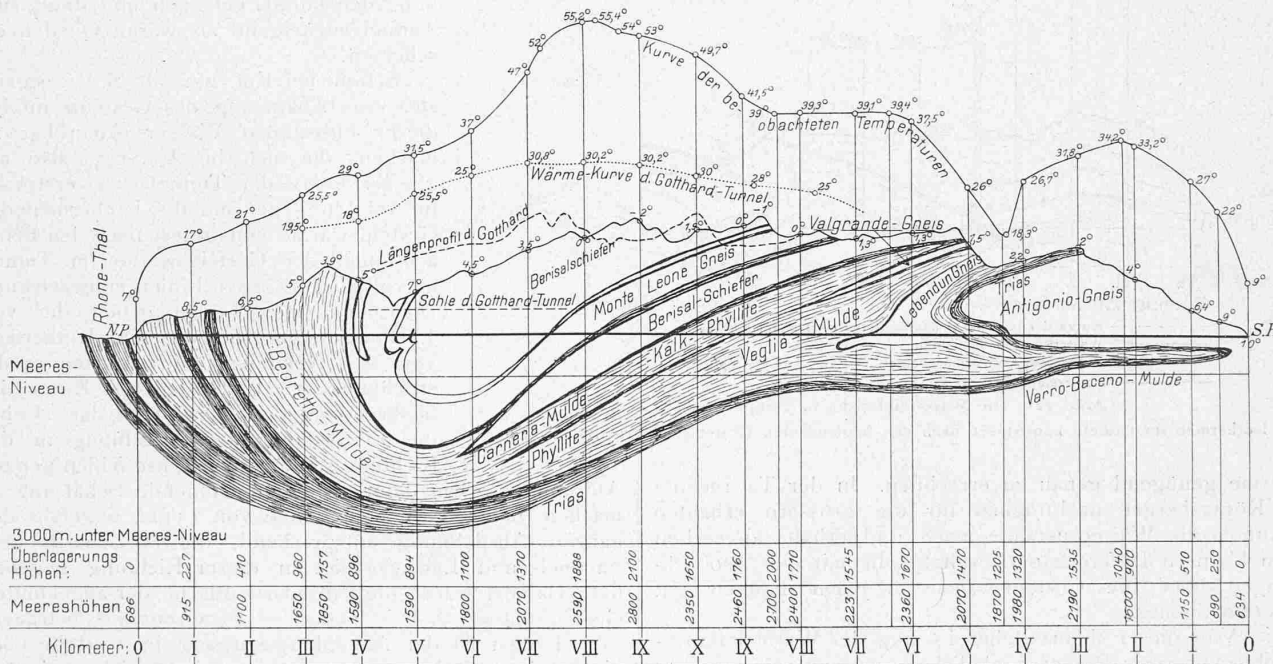
Abb. 21. Profil längs der Achse des Simplontunnels (Einpunktiert Gotthardtunnel) und geologisches Profil. — 1 : 120 000. Wärmekurven für beobachtete Temperaturen beim Simplontunnel und beim Gotthardtunnel. (Geologisches Profil gezeichnet nach dem von den Herren Schmidt und Preiswerk aufgestellten Profile.)
