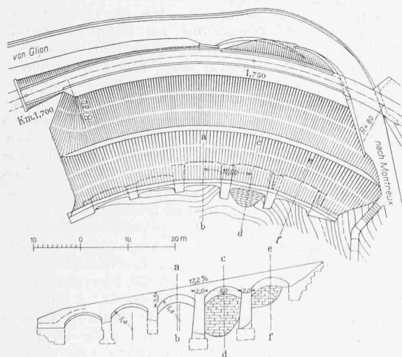
Abb. 20 und 21. Lageplan und Ansicht (1:1000) und Schnitte (1:300) der Lehengalerie in Abb. 22 für die Tunneldeponie.
