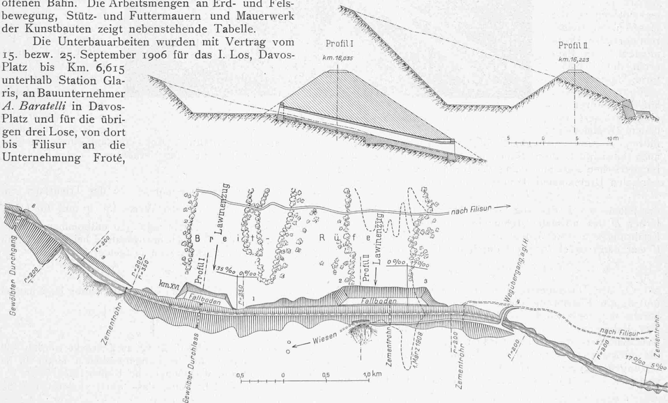
Abb. 20 und 21. Lawinen-Fallböden im Breitrüfzug. — Lageplan 1:4000, Querprofile 1:500.
