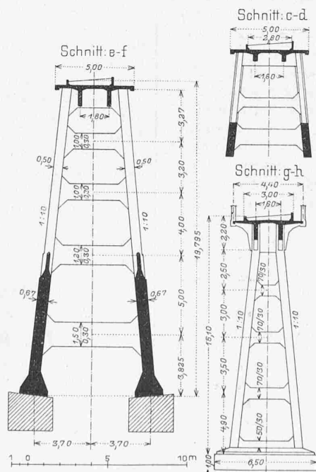
Abb. 4. Schnitte zu Abb. 3. — Massstab 1:300.
