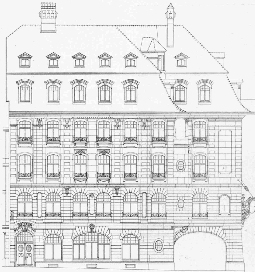
Abb. 6. Fassade an der Amtshausgasse. — Masstab 1 : 200.
