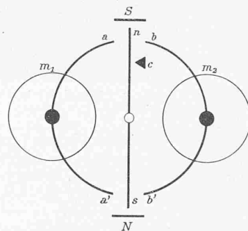
Abb. 5. Schema des Relais R_1 .
