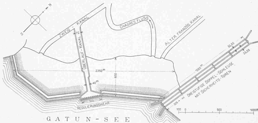
Abb. 6. Lageplan des Gatun-Dammes. — 1:30 000.
