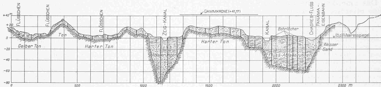
Abb. 5. Geologisches Profil längs der Gatun-Talsperre. — Masstab f. d. L. 1:15 000, f. d. Höhen 1:3500.
