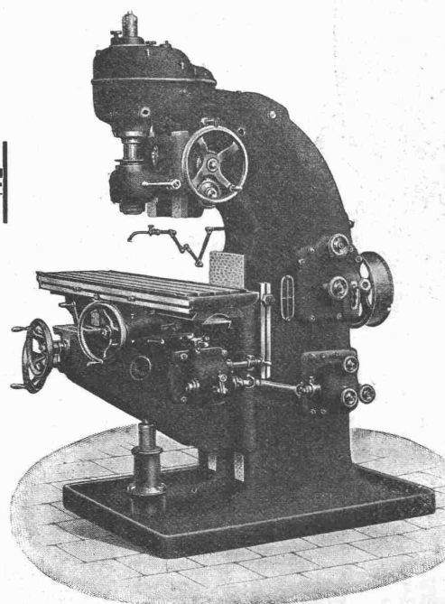
Vertikal-Fräsmaschine Nr. 3.
