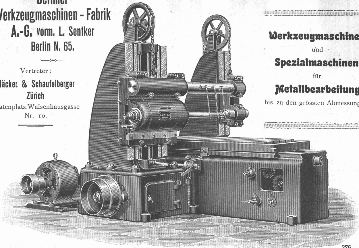
Langfraismaschine.
