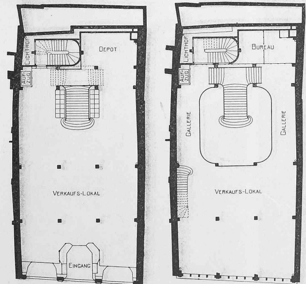
Abb. 5, 6, 7. Grundrisse vom Erdgeschoss, ersten und dritten Obergeschoss des Geschäftshaus G. Kiefer & Cie. — Masstab 1 : 400.
