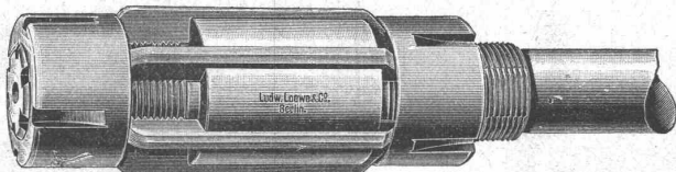
Nachstellbare Reibahle.
