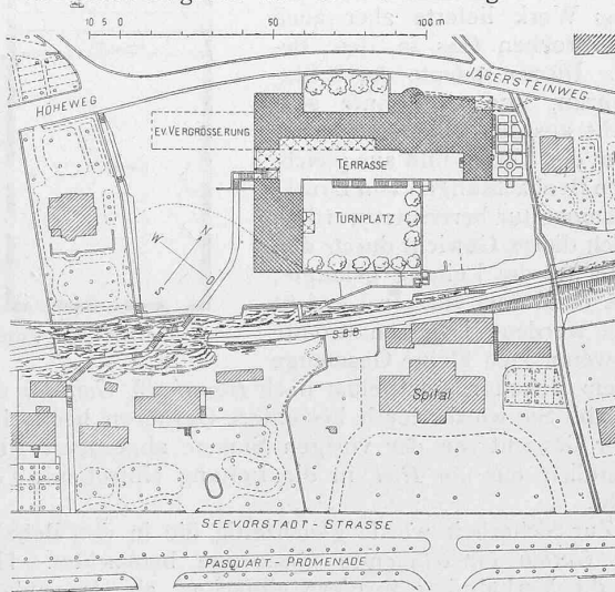
Lageplan. — Masstab 1 : 2500.
