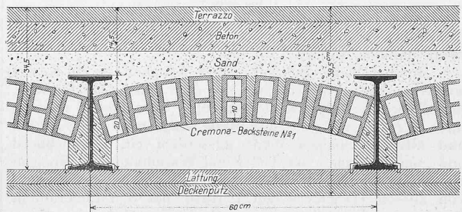
Abb. 11 und 12. Boden- und Deckenkonstruktionen über dem Erdgeschoss. — Masstab 1 : 10.
