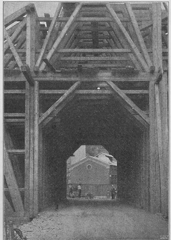
Abb. 12. Durchfahrt unter dem Lehrgerüste.
