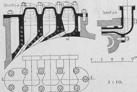
Abb. 2. Düsenapparat.
