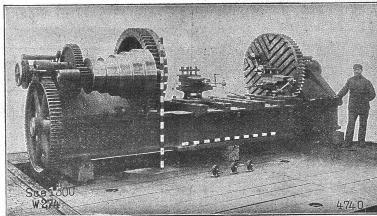
Radsatz-Drehbank.
