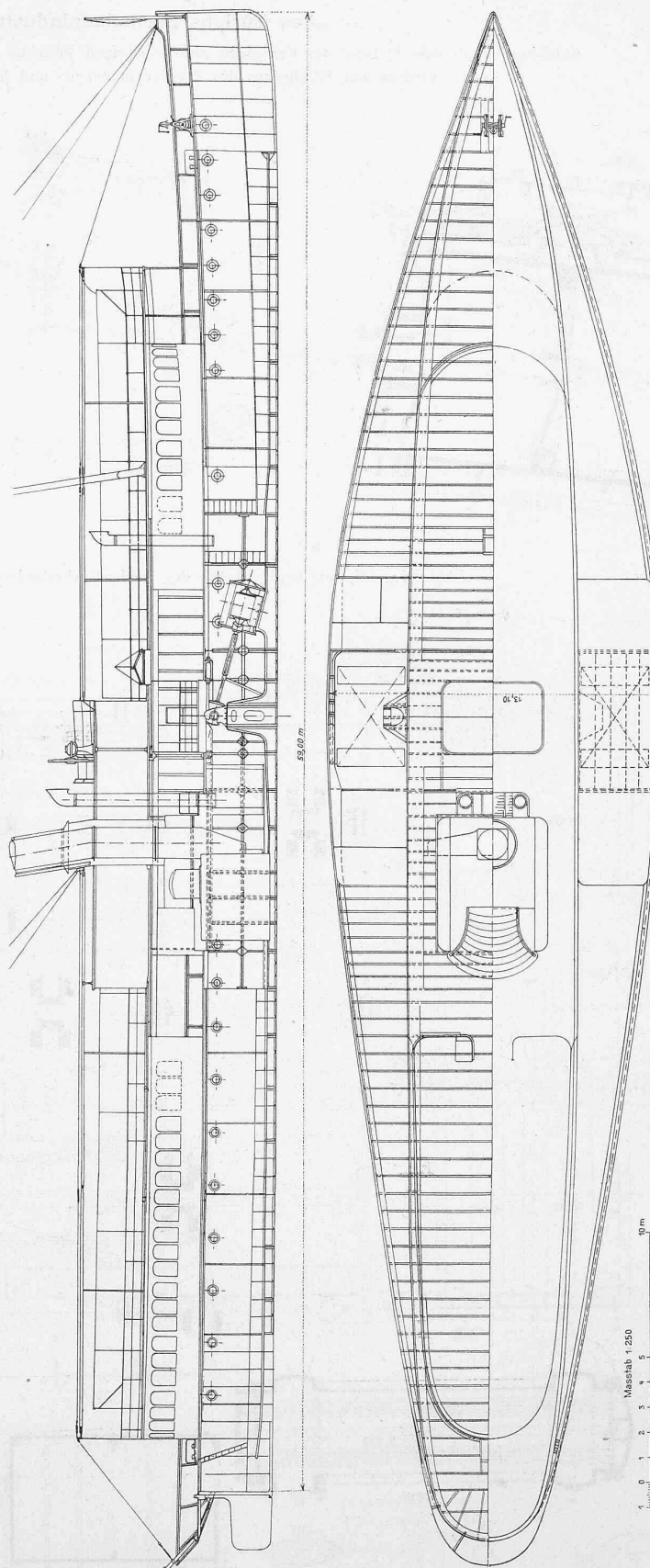
Abb. 5. Dampfboot «Unterwalden» mit 700 P. S. Verbundmaschine, für den Vierwaldstättersee gebaut von Escher Wyss & Cie. 1900. Längsschnitte und Grundriss. — Masstab 1:250.
