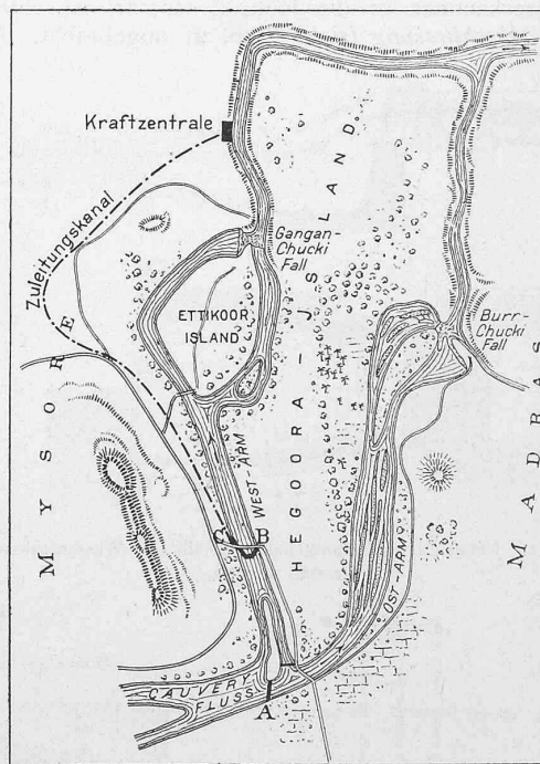
Abb. 1. Uebersichtsplan der ganzen Anlage. — 1:75000.
