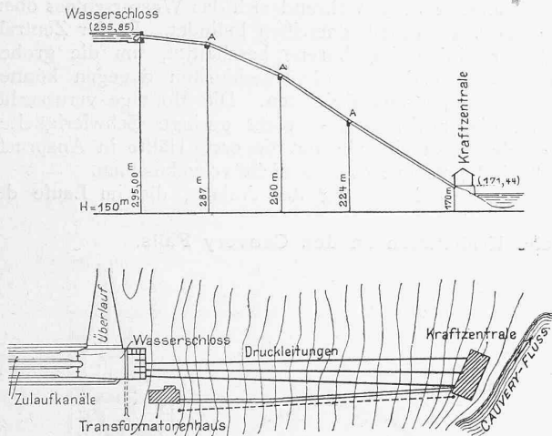
Abb. 8. Längenprofil und Lageplan der Druckleitung. Masstab 1:5000.
