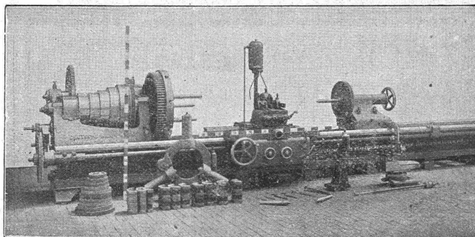
Transmissions-Wellen-Drehbank.
