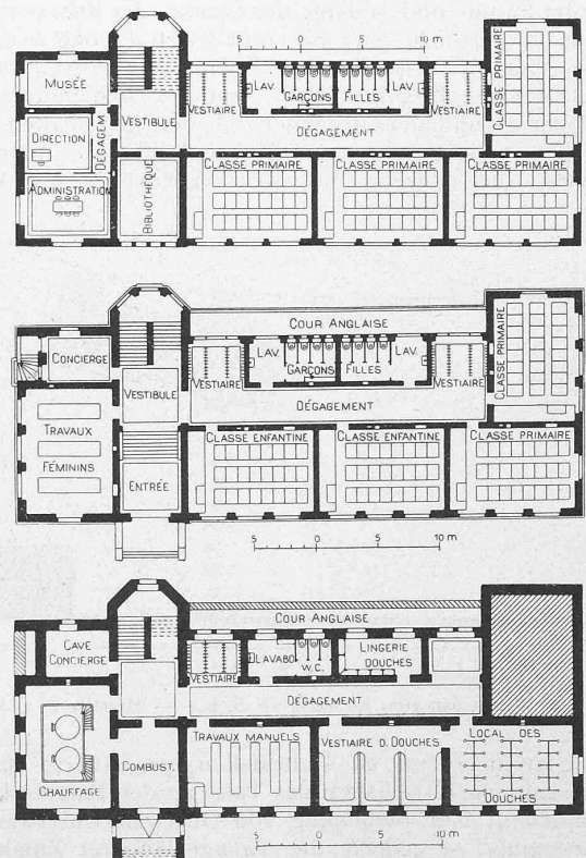
Grundrisse vom Untergergeschoss, Erdgeschoss und I. Stock. — 1 : 600.
