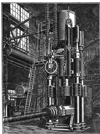
Dampfhdraulische Schmiedepresse. Stahlformguss bis zu 50 000 kg Stückgewicht.
