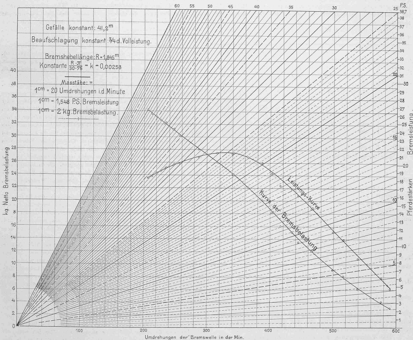
Graphische Rechentafel fur Bremsversuche von Prof. Dr. F. Prasil . — Masstab: 0,6 der nat. Grosse.
