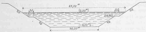
Abb. 4. Normalprofil in leichtem Terrain. — 1 : 1000.
