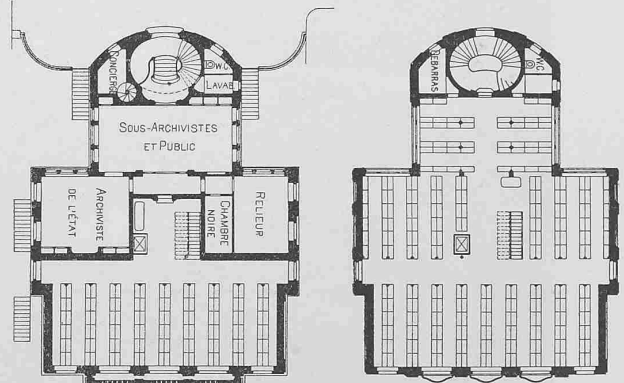
Grundriss vom Erdgeschoss. — 1 : 500. — Grundriss vom Obergeschoss.
