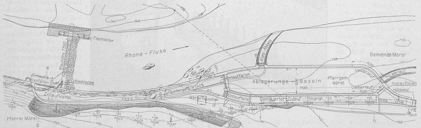
Abb. 7. Lageplan von Wehr, Einlaufkanal und Ablagerungsbassin. — Masstab 1 : 1000.
