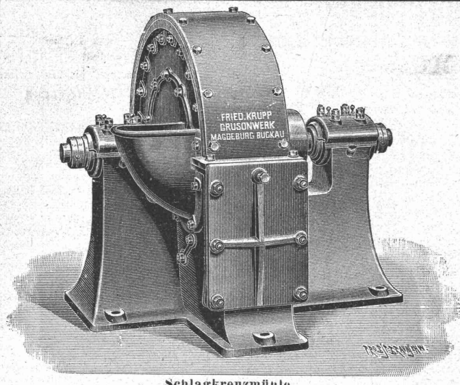
Schlagkreuzmühle.
