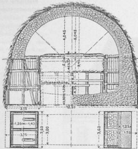
Fig. 6. Ausführung des zweigleisigen Tunnels in wenig drückendem Gebirge.
