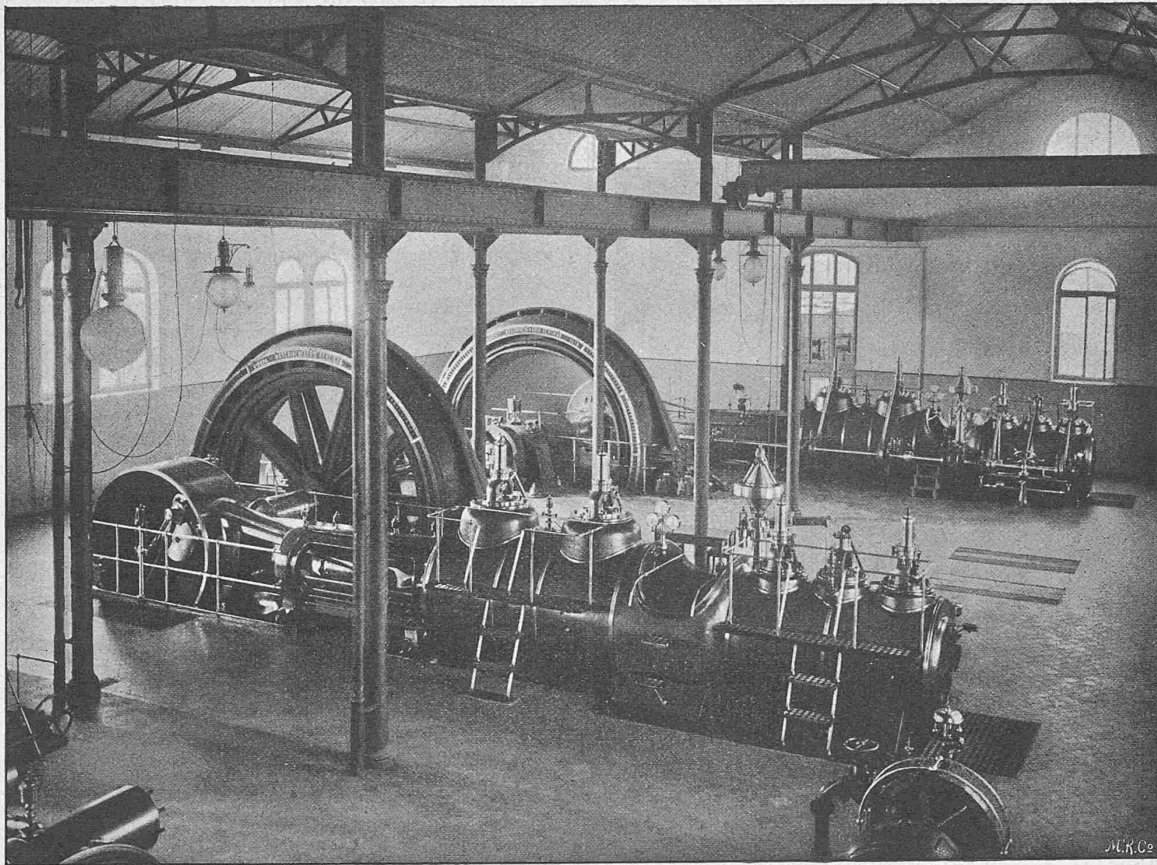
Fig. 3. Maschinenaal. — Ansicht der 1000 P. S.-Ventildampfmaschinen.
