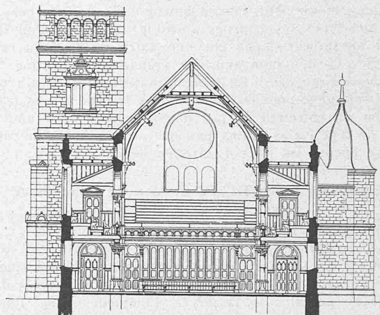
Querschnitt 1:300.
