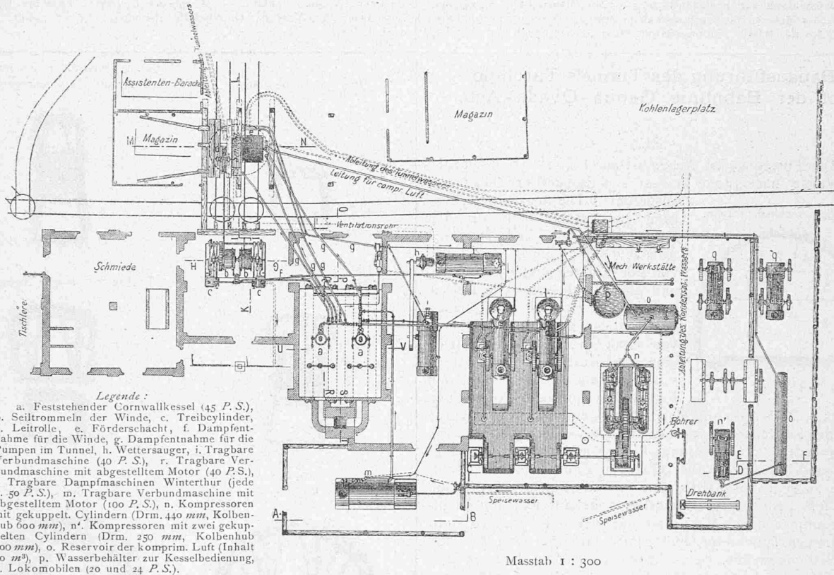
Fig. 11. Anlagen und Einrichtungen an der Baustelle.
