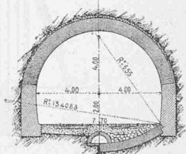
Fig. 10. Fertiger Tunnel ohne mit Sohlengewölbe.
