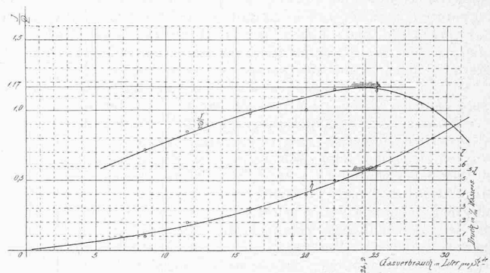
Fig. 3. Wirkungsgrade des Brenners Patent Billwiller.
