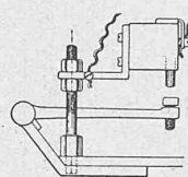
Fig. 7. Kontakt-Vorrichtung.
