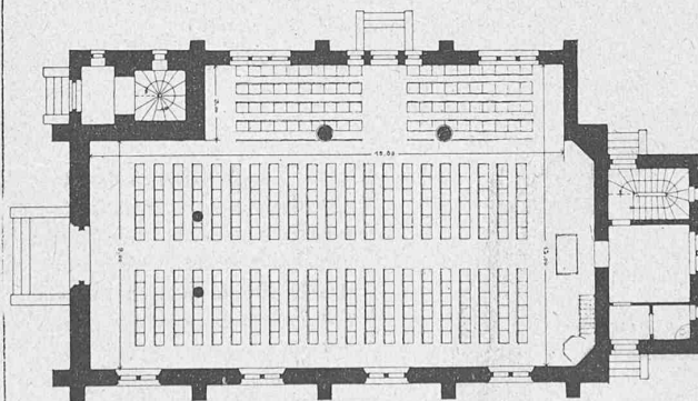
Hauptgrundriss. 1 : 300.
