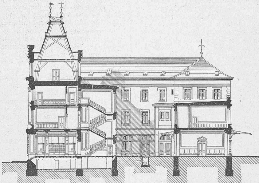
Schnitt.
