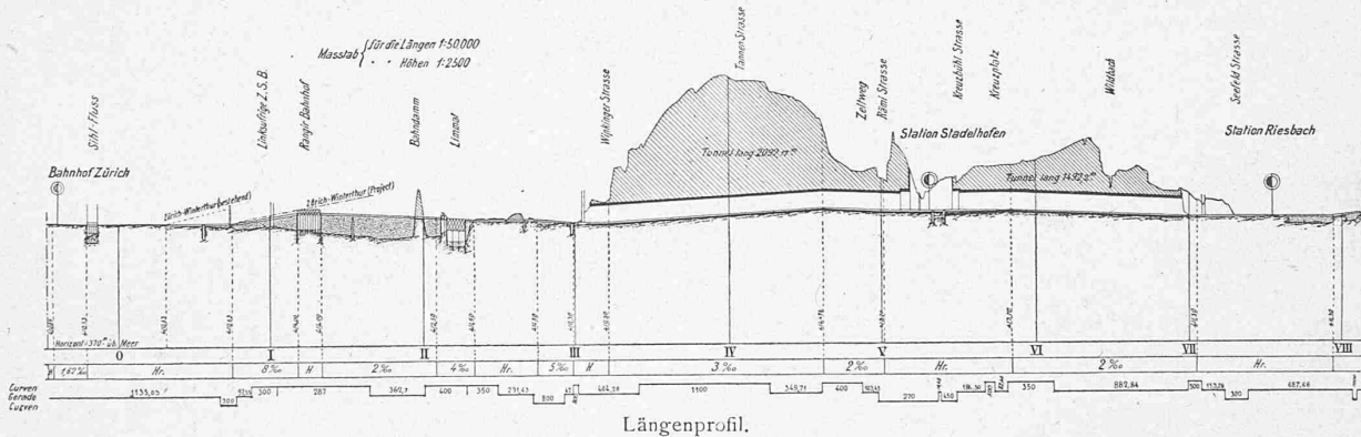
Längenprofil.
