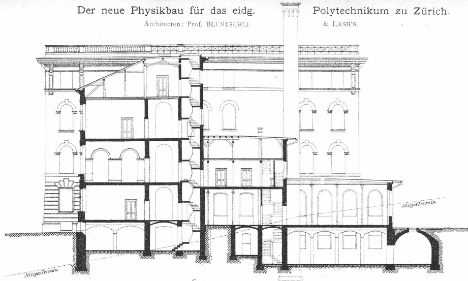
SCHNITT G-H.
