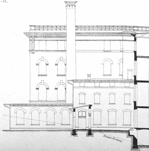
SCHNITT C-D.
