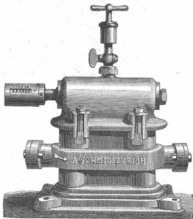
Bewährter Wassermesser zur Controle der Dampfkessel. (M 1474 Z) Medaille d'honneur de la Société industrielle de Mulhouse 1885.
