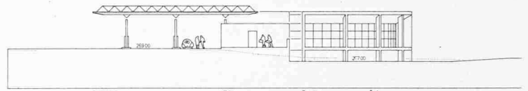
Buvette Westansicht 1:700
