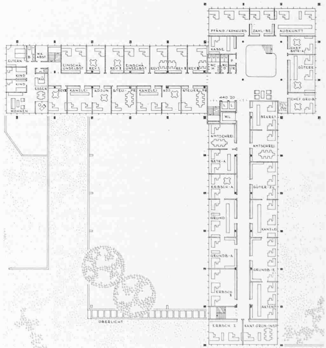
Unten rechts: Grundriss 2. Obergeschoss 1:750 (2. Stufe, Bearbeitungsgrad 1:200)
